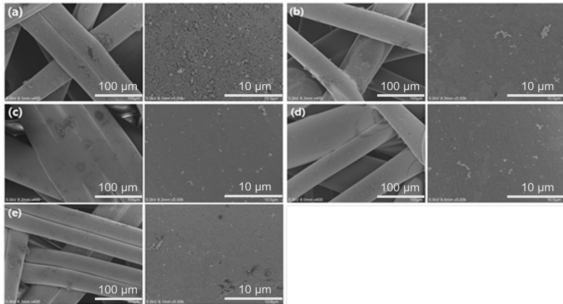
Figure 2. FE-SEM photographs: PP filter with Ag ELP for (a) 1 min, (b) 2 min, (c) 3 min, (d) 4 min, and (e) 5 min.
