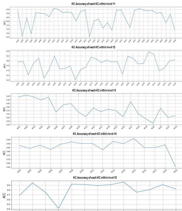
그림 3. 레벨별 KC 정확도의 평균 그래프
