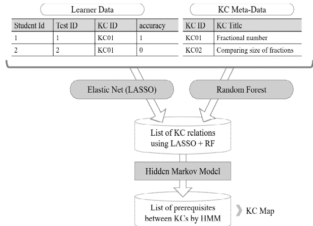
그림 2. LASSO + RF + HMM 모델의 구조 Fig. 2. Structure of LASSO + RF + HMM model
