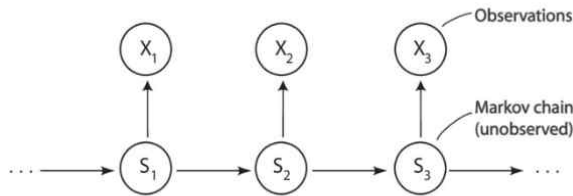
그림 1. HMM과 관측치 Fig. 1. HMM and its observations
